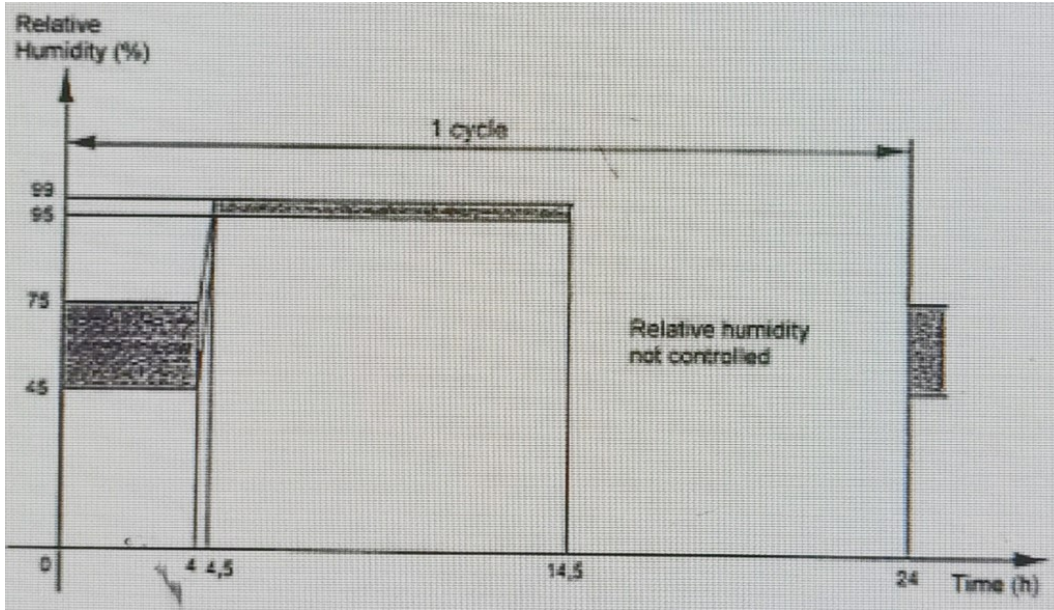
图 10. 温湿度循环
