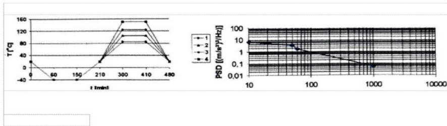
图 8.随机振动测试中的温度循环规格
