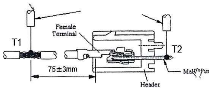
图 4. 接触电阻测试方法
