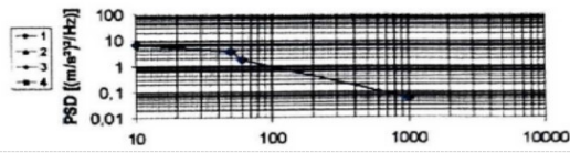
图 9.Body(弹性质量)随机振动表
