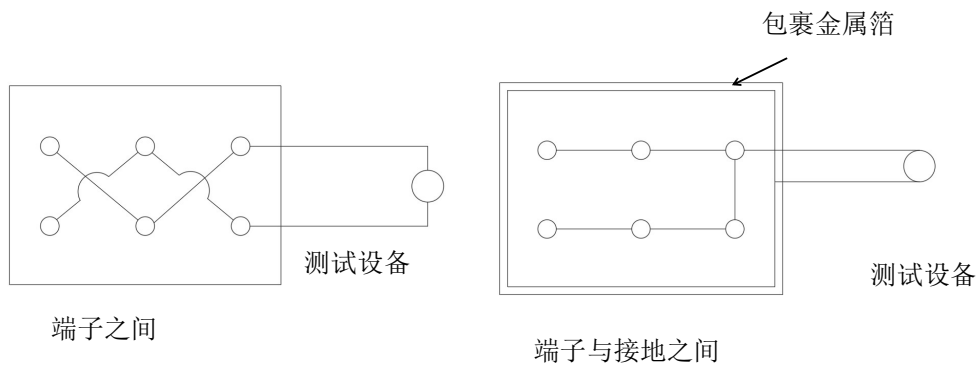
图 6. 绝缘电阻测试方法
