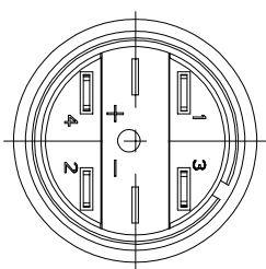
焊接面视图
