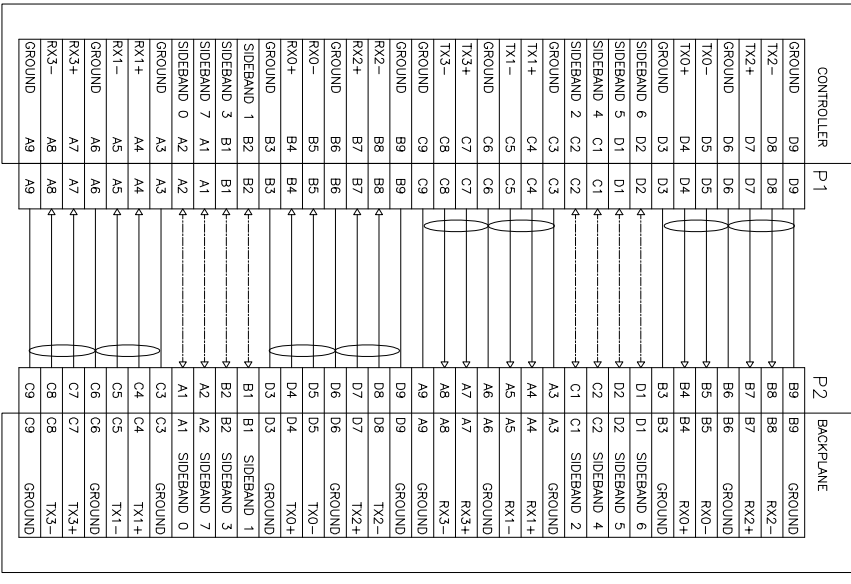
WIRING TABLE
